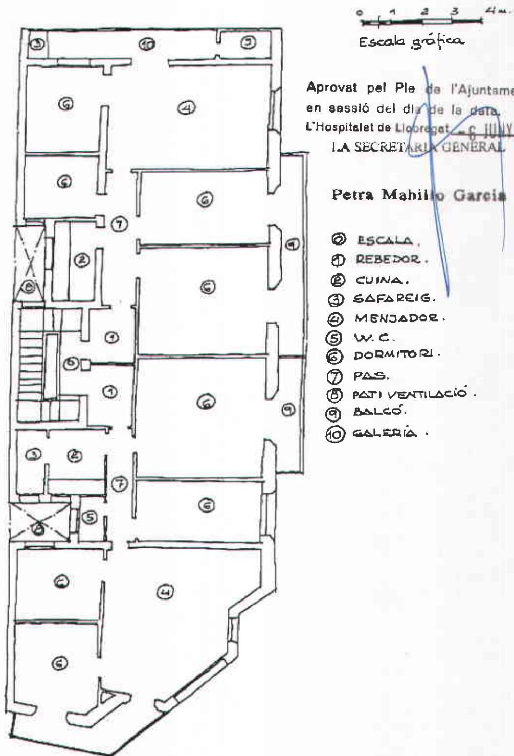
Planta tipus segons PEPPA
